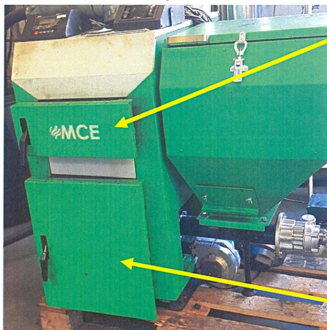
Kocioł c.o. „V6” o mocy 8 kW
