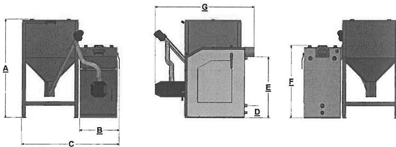
Rysunek 2 Wymiary kotła
