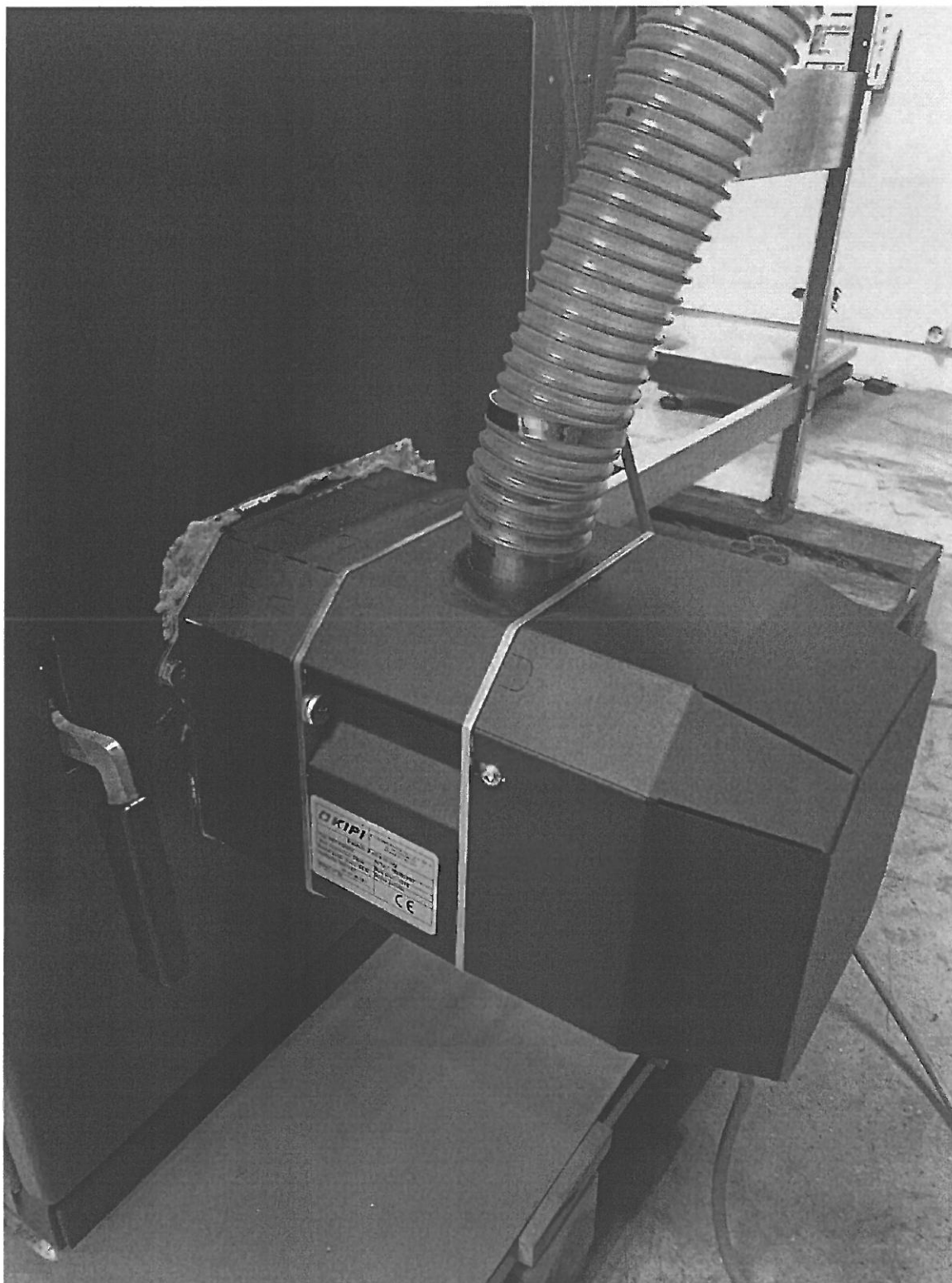
Rysunek 5 Palnik KIPi
