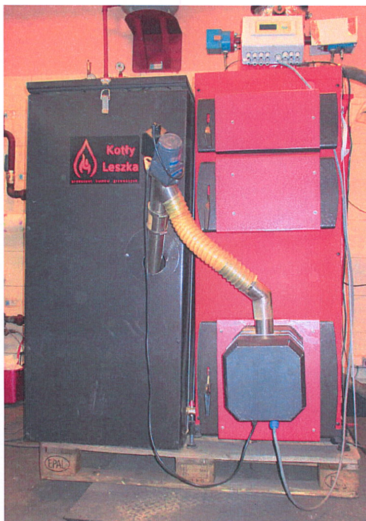
Rysunek 1. Fotografia kotła KATLA
