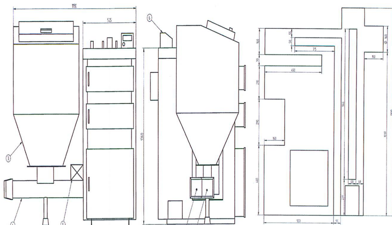
Rysunek 2. Schemat konstrukcyjny i gabaryty kotła HEKLA
