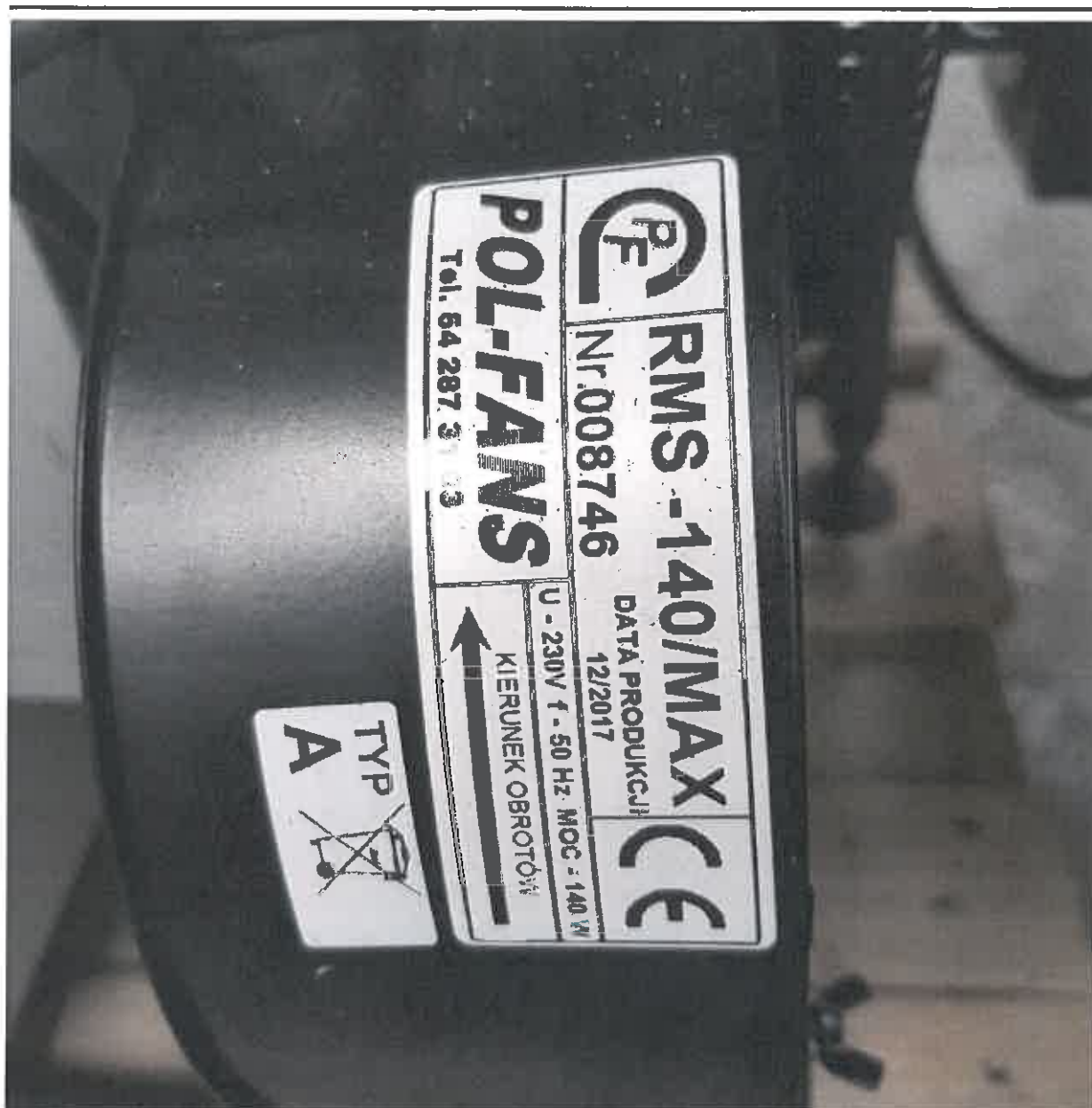
Rysunek 12 Dmuchawa RMS-140/MAX firmy POL-FANS
