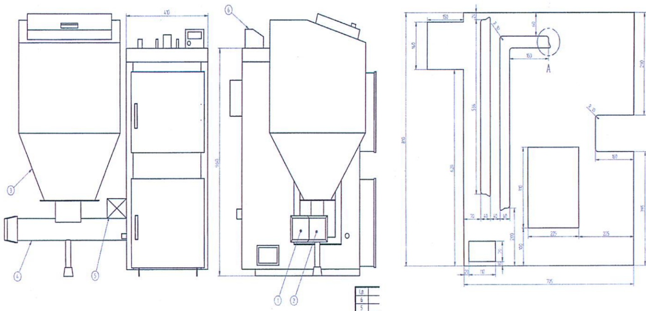
Rysunek 2. Schemat konstrukcyjny i gabaryty kotła HEKLA
