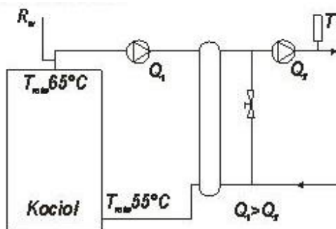
Rys. 8 Schemat połączenia kotła z instalacją grzewczą z wykorzystaniem sprężki wodnego.
