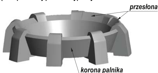
Rysunek 12. Wygląd korony palnika retortowego /na przykładzie APPS 15 kW/.
