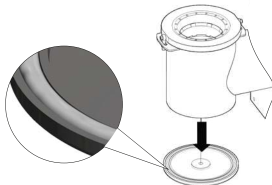
KROK 2. Zdjąć dekiel wyczystki palnika retortowego, oczyścić korpus palnika, sprawdzić stan sznura uszczelniającego.
