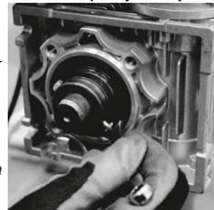
Krok 6. Zabezpieczyć śrubę nakrętką
