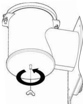
KROK 1. Odkręcić nakrętkę motylkową mocującą dekiel wyczystki palnika retortowego.
