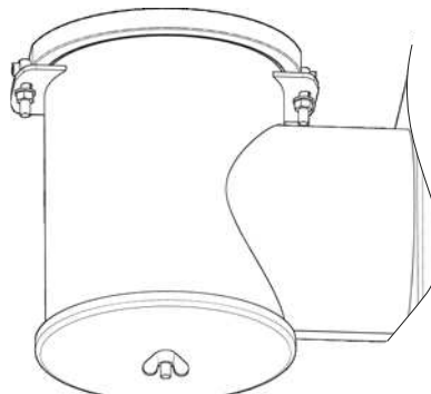
KROK 3. Zamontować szczelnie dekiel wyczystki przykręcając go nakrętką motylkową. Powyżej zamontowana wyczystka palnika retortowego
