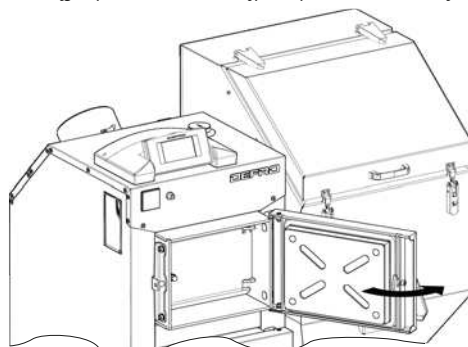
KROK 1. Otworzyć drzwi wyczystne.
