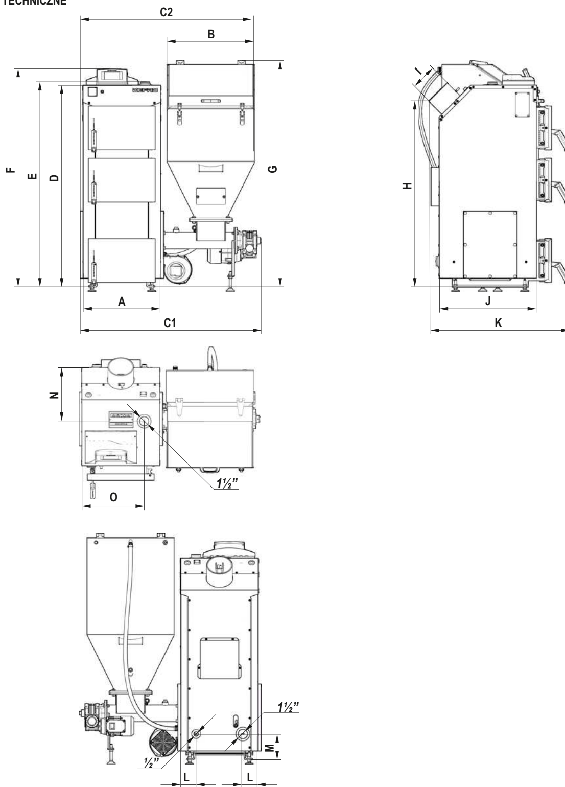
Rysunek 1. Podstawowe wymiary kotłów KOMFORT EKO MINI.
