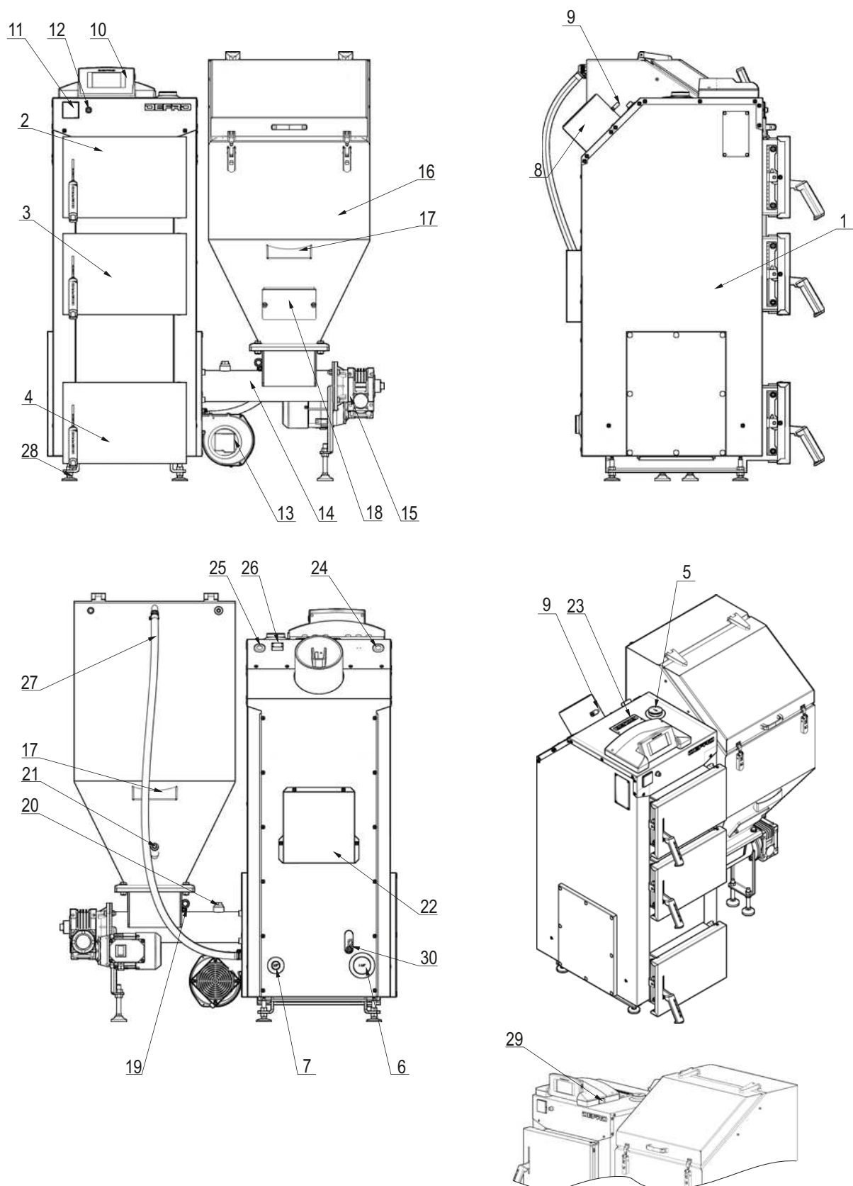
Rysunek 2. Podstawowe elementy kotłów KOMFORTEKO MINI.
