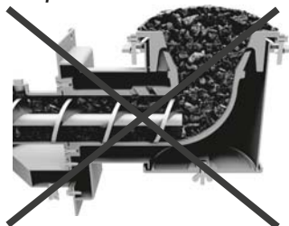
Rysunek 15. Prawidłowy wygląd paleniska przy spalaniu węgla.
