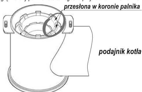
Rysunek 13. Prawidłowe położenie korony palnika retortowego.
