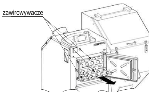
KROK 3. Ostrożnie wysunąć zaworowycze i oczyścić.
