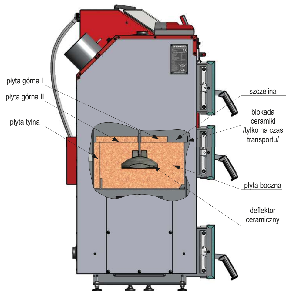
Rysunek 24. Rozmieszczenie katalizatorów ceramicznych w kotle.
