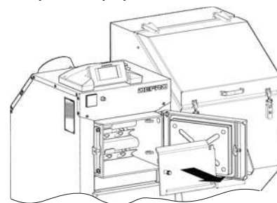
KROK 2. Ostrożnie unieść, lekko przechylić i zdjąć z zawiasów drzwi odbojnicowe, a następnie wyjąć je z kotła.
