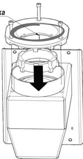
KROK 5. Zmontować palnik retortowy zwracając uwagę, aby przesłony znajdowały się na wprost rury podawczej podajnika.
