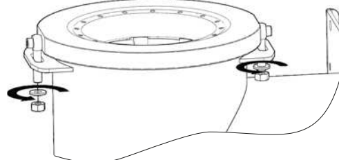
KROK 1. Odkręcić nakrętki mocujące płytę palnika retortowego.
