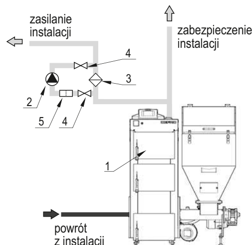
Rysunek 9. Wykonanie obejścia grawitacyjnego: 1-kocioł; 2-pompa obiegowa; 3-zawór różnicowy; 4-zawory odcinające; 5-filtr; 6-otwarte naczynia wzbiorcze.
