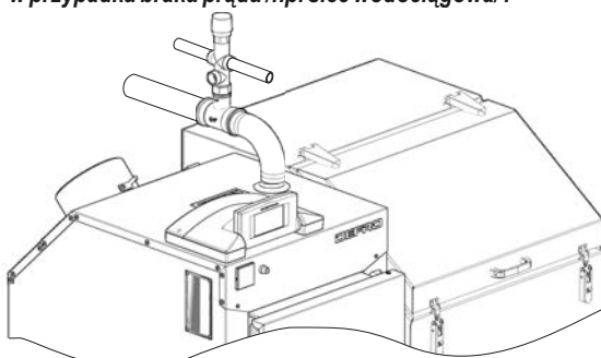
Rysunek 8. Przykładowy sposób podłączenia zaworu DBV-2.
