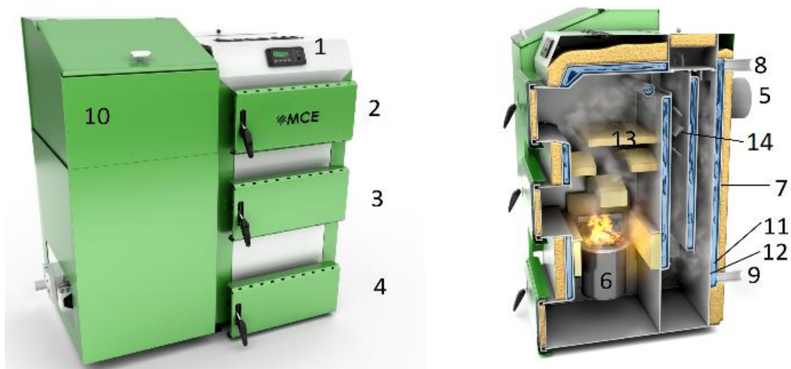
RYS. 2. PRZEKRÓJ KOTŁA V6 16 I V6 20
