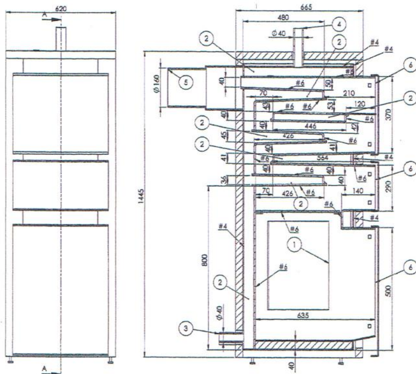
Rysunek 2. Schemat konstrukcyjny i gabaryty kotła TECHNIX
