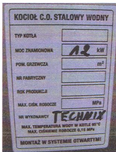
Rys. 2. Tabliczka znamionowa kotła typu Technix 12.
