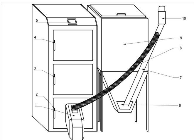
Rys.1 Schemat konstrukcji kotła VIP Pellet 20-35
