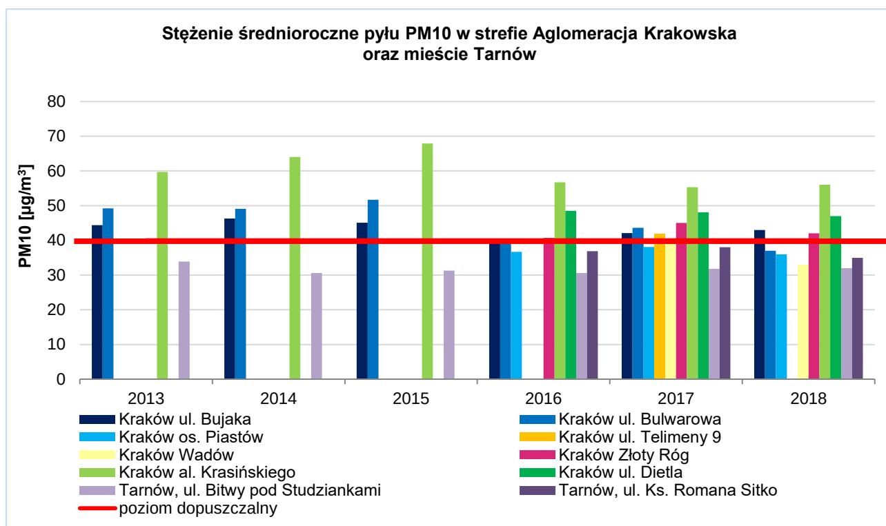
Rysunek 2. Stężenia średnioroczne pyłu PM10 w strefach Aglomeracja Krakowska oraz miasto Tarnów. 8
