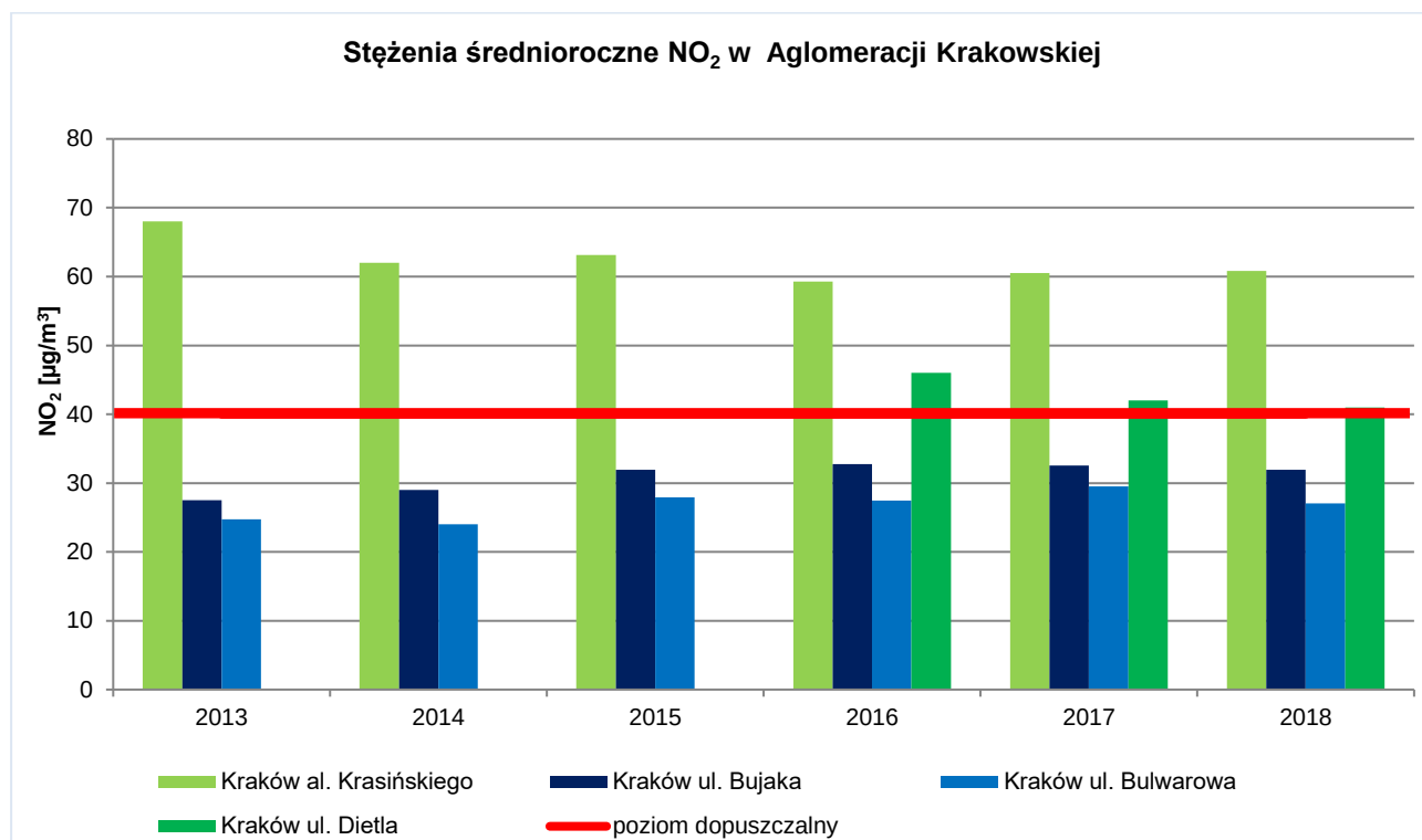
Rysunek 7. Wartości stężeń średniorocznych dwutlenku azotu w Aglomeracji Krakowskiej na stacjach monitoringu jakości powietrza 14 .
