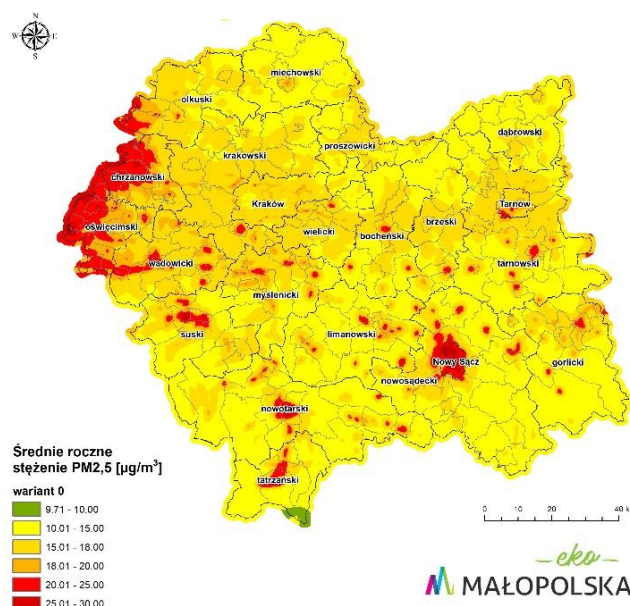
Rysunek 17. Średnioroczne stężenie pyłu PM2,5 w roku prognozy 2023 w przypadku niepodjęcia systemowych działań i przy zachowaniu obecnego trendu działań naprawczych 32 .
