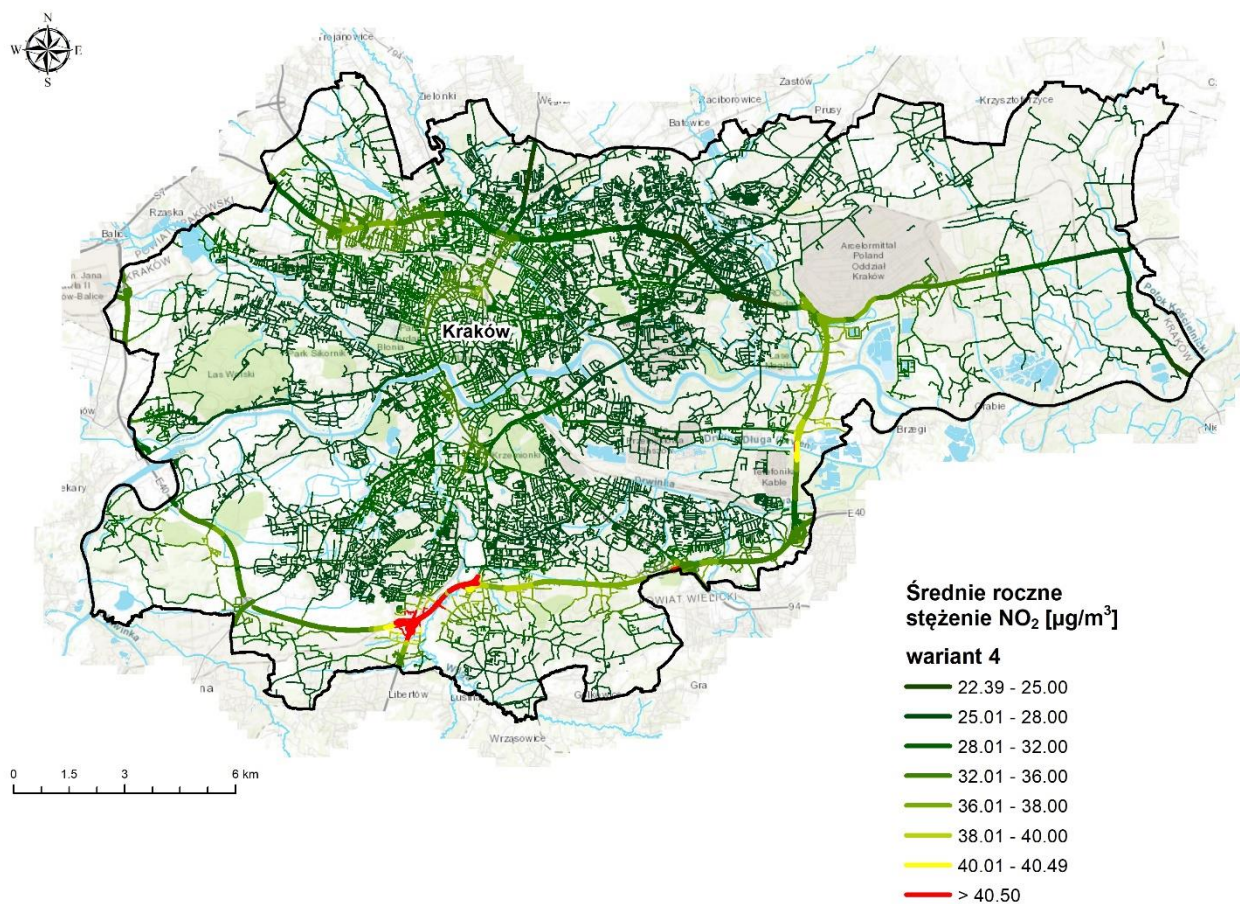
Rysunek 30. Rozkład oczekiwanych stężeń średniorocznych dwutlenku azotu w Aglomeracji Krakowskiej w 2026 r. 77
