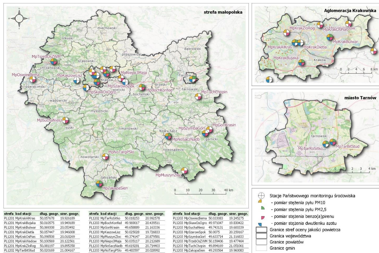
Rysunek 1. Lokalizacja stref ochrony powietrza i stacji pomiarowych w województwie małopolskim wykorzystywanych w rocznej ocenie jakości powietrza za rok 2018 7 .
