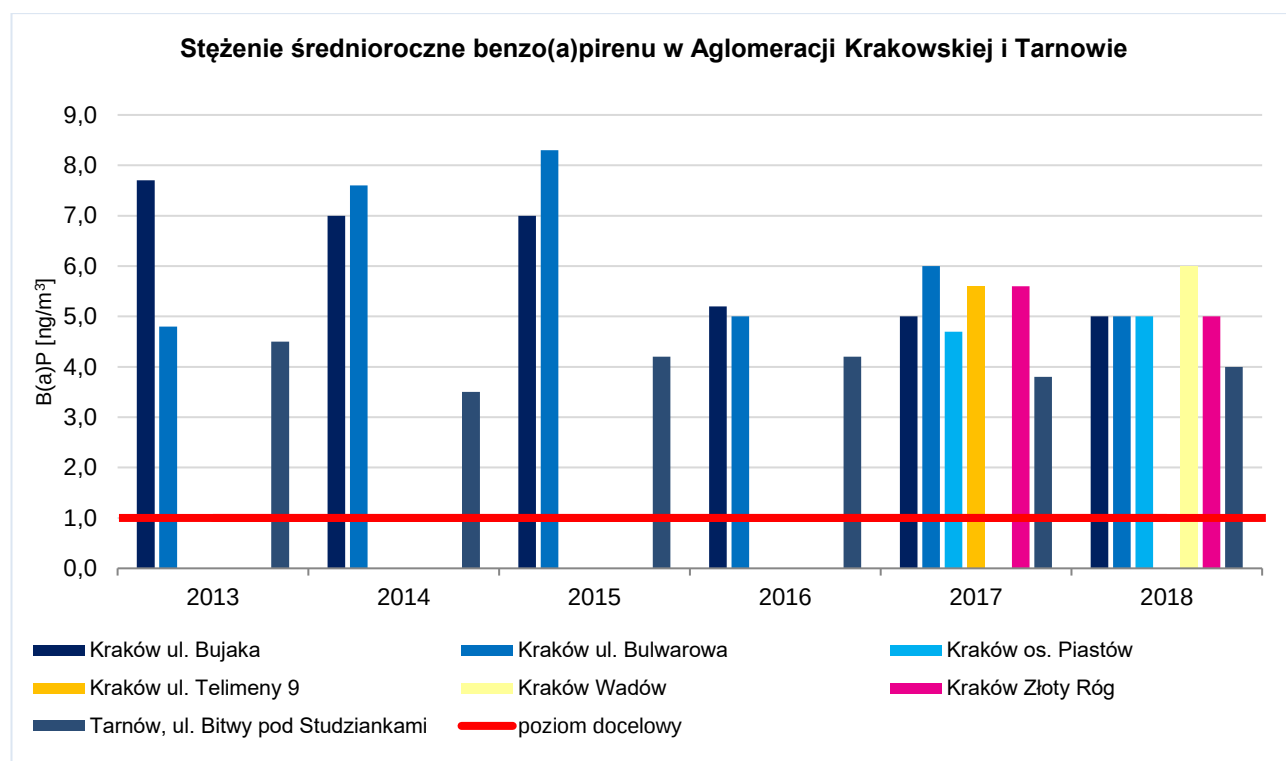
Rysunek 5. Wartości stężeń średniorocznych benzo(a)pirenu na stacjach monitoringu jakości powietrza w Aglomeracji Krakowskiej i Tarnowie 12 .
