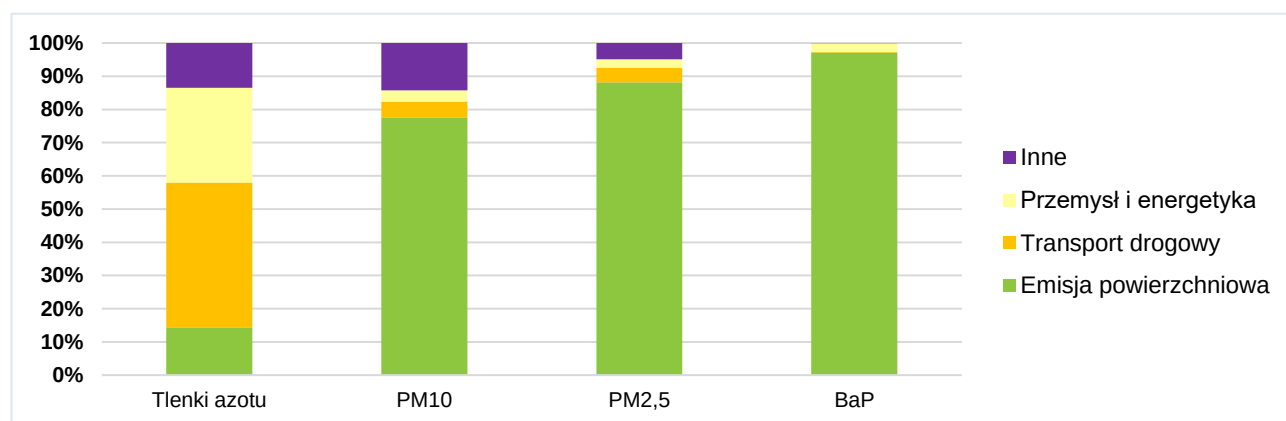
Rysunek 20. Wielkości emisji pyłu PM 10 , PM 2,5 , benzo(a)pirenu i dwutlenku azotu w podziale na rodzaje źródeł w województwie małopolskim w 2018 r. 36
