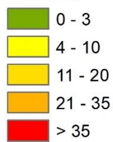
Rysunek 27. Rozkład ilości dni z przekroczeniem normy dobrego pyłu PM10 w województwie małopolskim w 2023 r. 74
