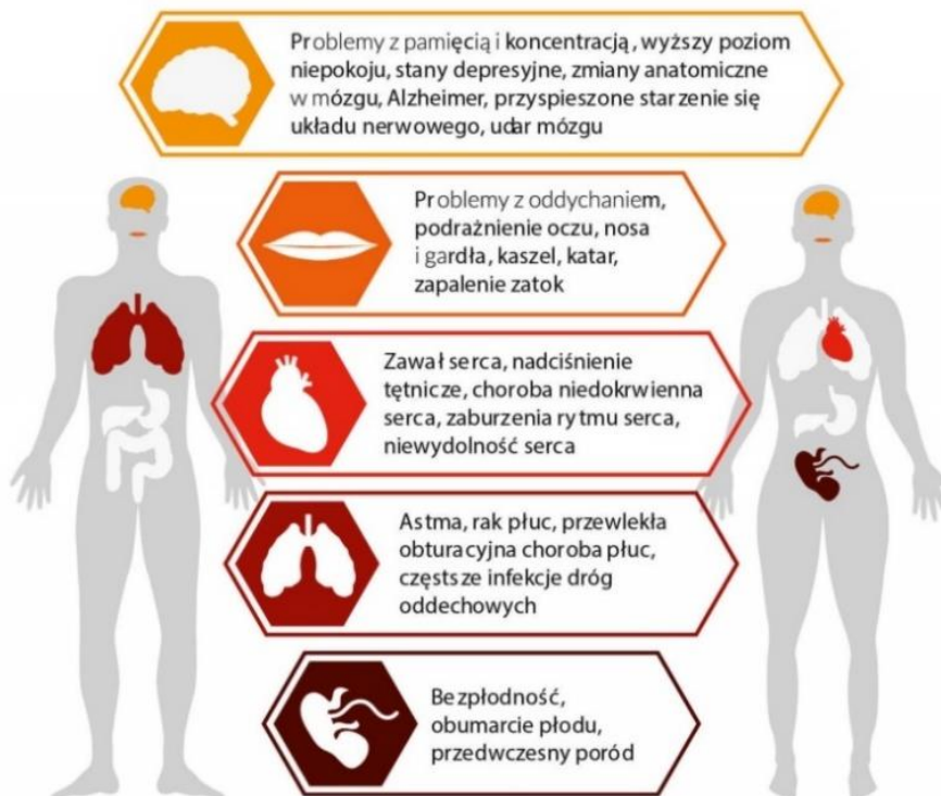
Rysunek 24. Wpływ zanieczyszczeń powietrza na zdrowie ludzkie 42
