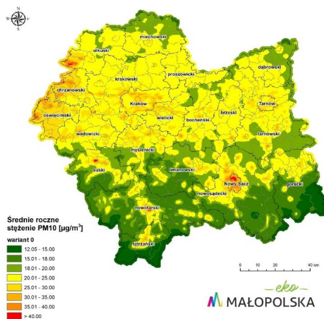
Rysunek 16. Średnioroczne stężenie pyłu PM10 w roku prognozy 2023 w przypadku niepodjęcia systemowych działań i przy zachowaniu obecnego trendu działań naprawczych 31 .
