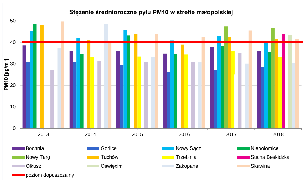
Rysunek 3. Stężenia średnioroczne pyłu PM10 w strefie małopolskiej 9 .
