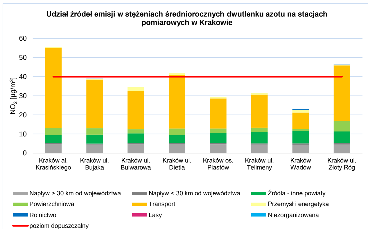
Rysunek 23. Udział źródeł emisji w stężeniach średniorocznych dwutlenku azotu na stacjach pomiarowych w Aglomeracji Krakowskiej w 2018 r. 39
