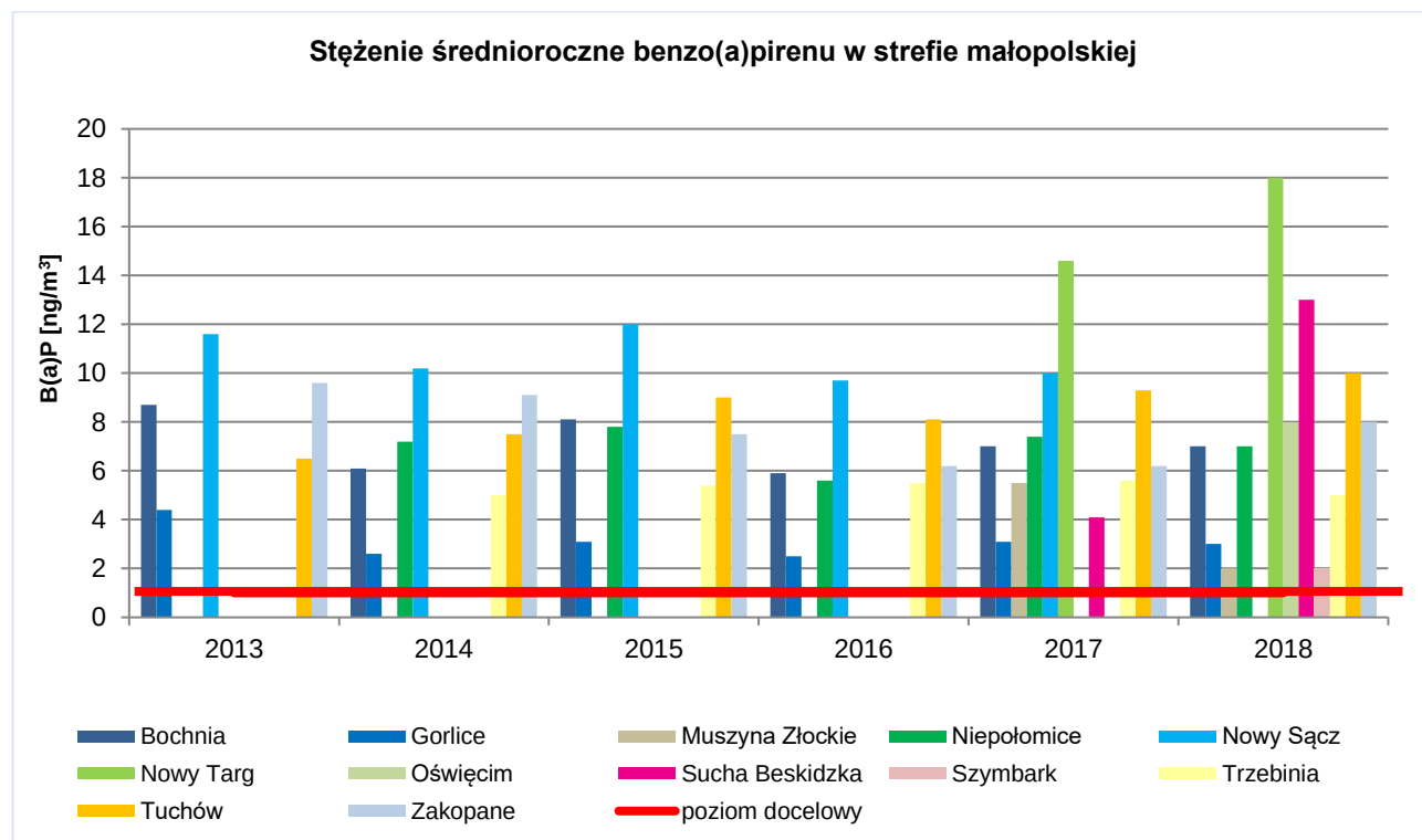
Rysunek 6. Wartości stężeń średniorocznych benzo(a)pirenu na stacjach monitoringu jakości powietrza w strefie małopolskiej 13 .
