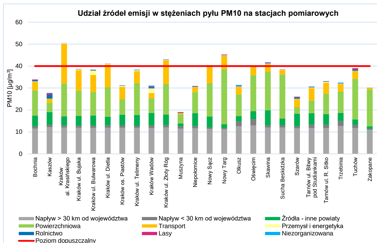
Rysunek 21. Udział źródeł emisji w stężeniach średniorocznych pyłu PM 10 na stacjach pomiarowych w województwie w 2018 r. 37
