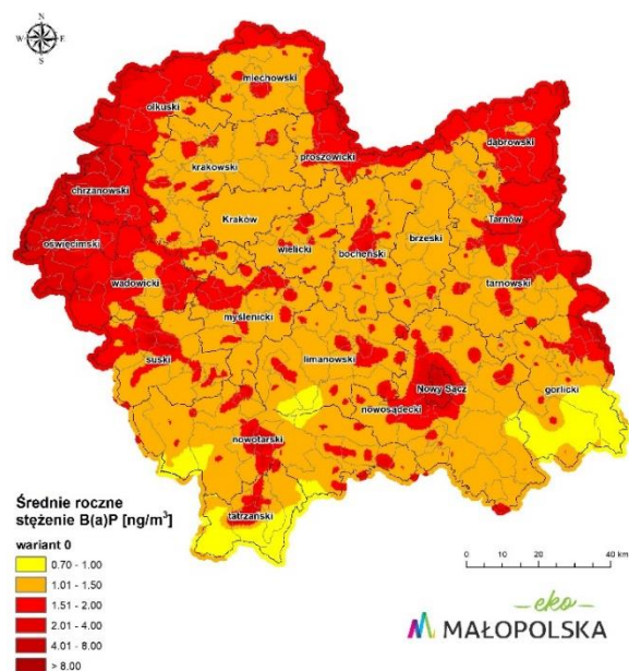
Rysunek 18. Średnioroczne stężenie benzo(a)pirenu w roku prognozy 2023 w przypadku niepodjęcia systemowych działań i przy zachowaniu obecnego trendu działań naprawczych 33 .
