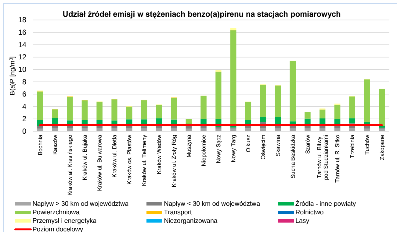
Rysunek 22. Udział źródeł emisji w stężeniach średniorocznych benzo(a)pirenu na stacjach pomiarowych w województwie w 2018 r. 38
