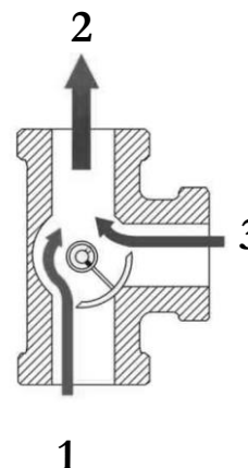
Rys. 10a. Przykład montażu zaworu mieszającego w instalacji z regulacją ilościową (zapewnia ochronę kotła przed „zimnym” powrotem czynnika grzewczego).
