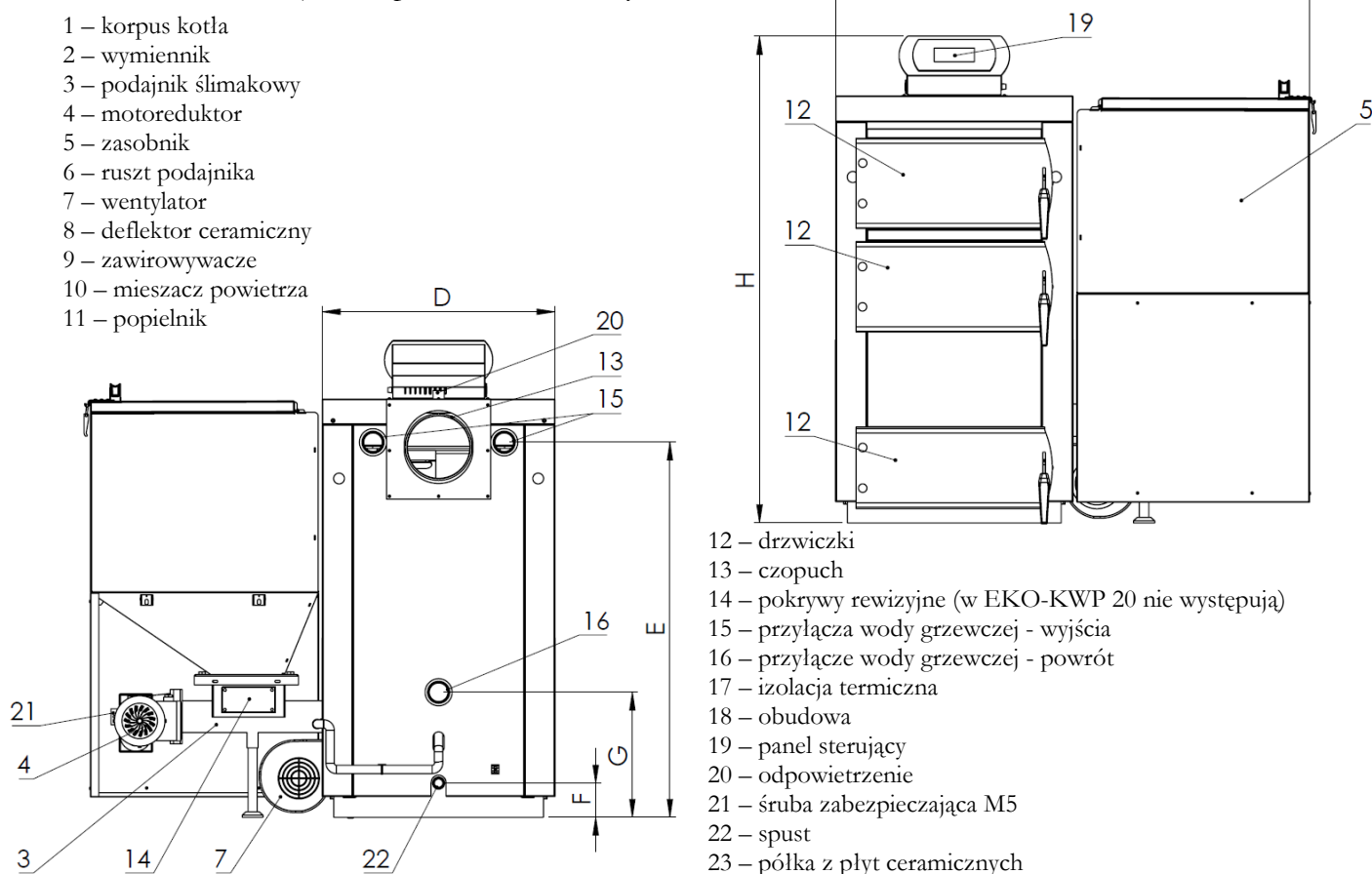
Rys. 1a. Konstrukcja i opis kotłów EKO-KWP
