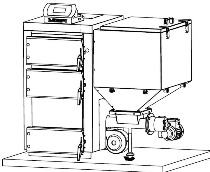
Rys. 7b. Późimowanie zasobnika kotła.
