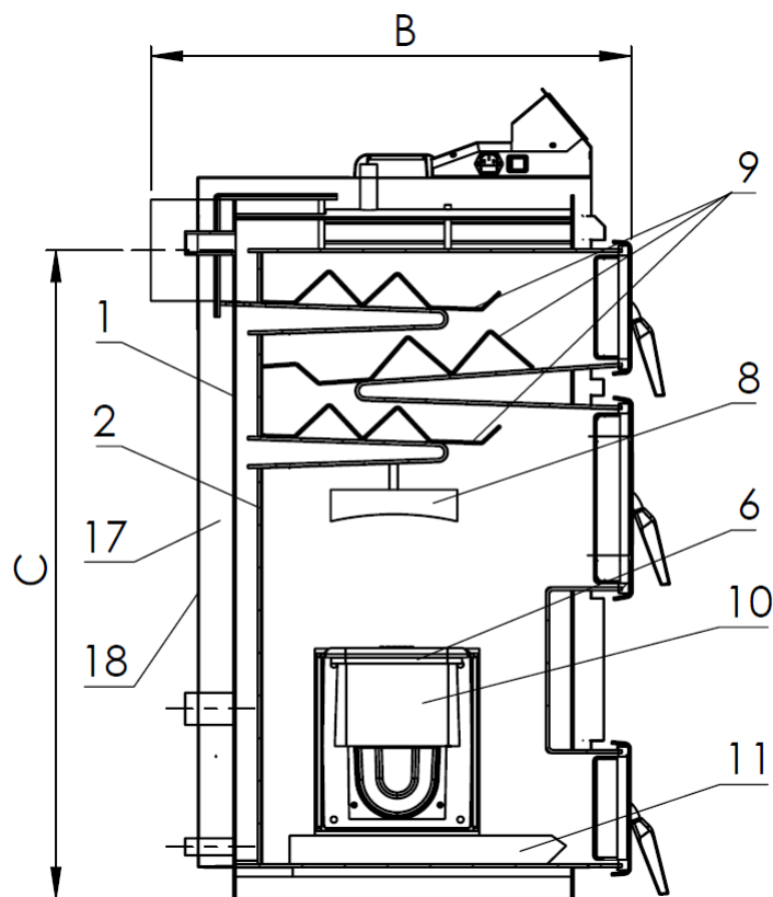
Rys. 1b. Konstrukcja i wymiary kotłów EKO – KWP 20
