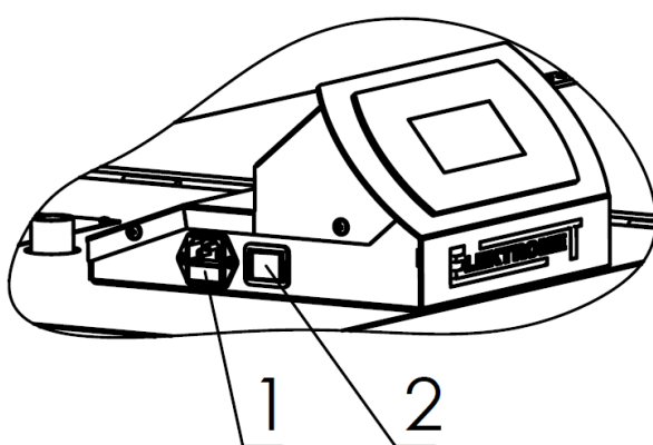
Rys. 3b Listwa przyłączy sterownika Estyma Compact KWP
