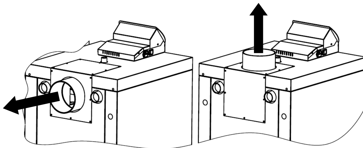
Rys.2 Możliwości montażu czopucha
