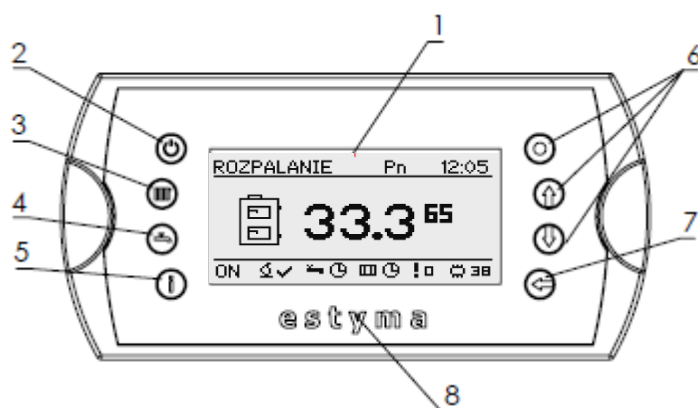
Rys. 3a Panel sterujący sterownika Estyma Compact KWP
