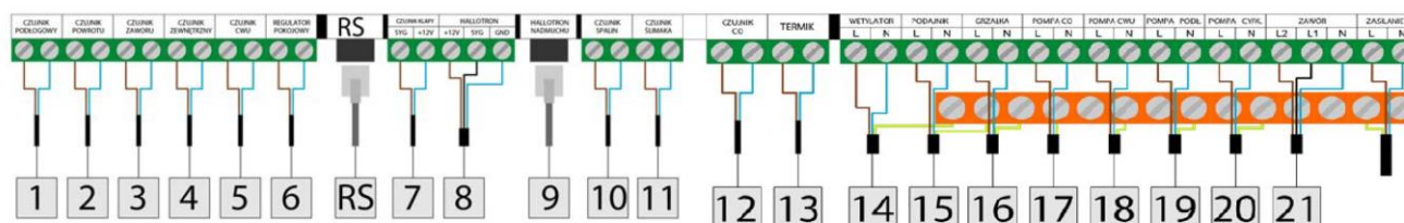
Rys. 4a Panel sterujący sterownika EL-683zPID.
