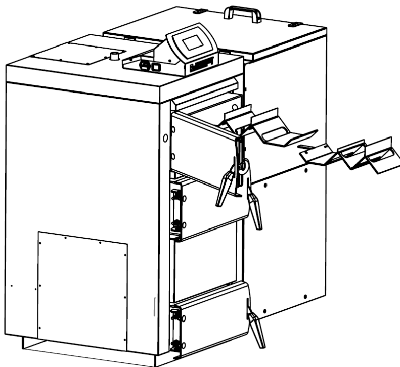
Rys. 12b. Demontaż zawirowywaczy spalin.
