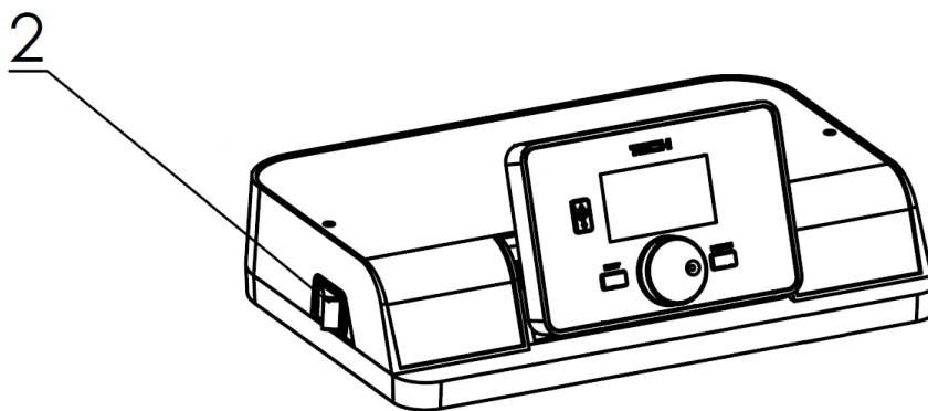
Rys. 12c. Umieszczenie głównego wyłącznika kotła.
