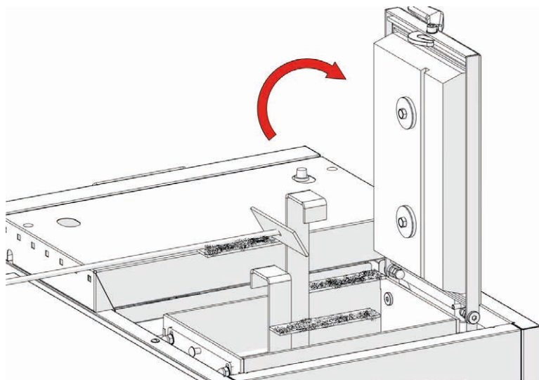
Rys. Zawirowywacze dla modelu 8, 10, 12, 24 kW
