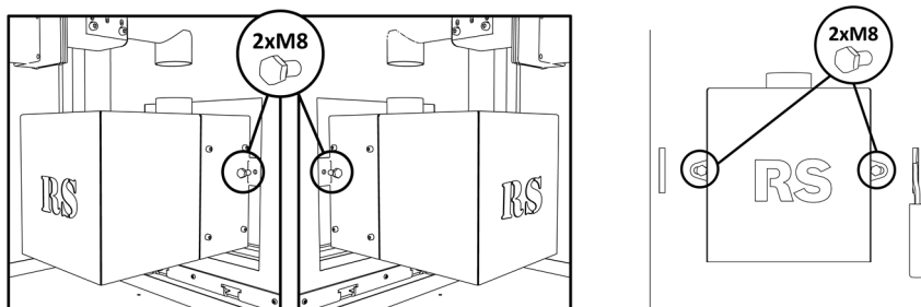
Rys. 14. Odkręcenie śrub mocujących palnik
