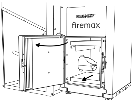
Rys. 10. Opróżnianie popielnika
