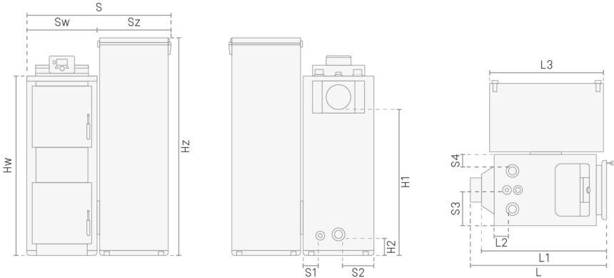
Rys. 4. Wymiary kotła Firemax 190 plus
