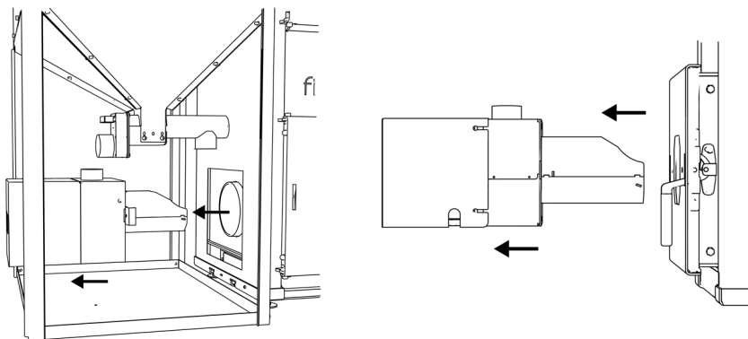
Rys. 15. Wyciąganie palnika
