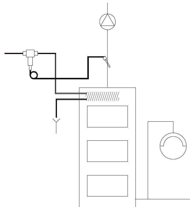
Rysunek 14.1 Schemat zabezpieczenia kotła za pomocą wbudowanej wężownicy chłodzącej i z zabezpieczeniem termicznym.
