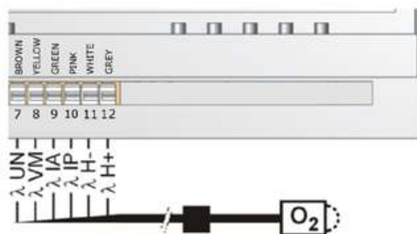
ecoLambda 2B - schemat podłączenia sondy Lambda.
