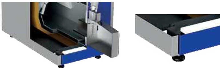
Rys. 2. Stopka regulacyjna, służąca do wypoziomowania kotła typu BIO COMPACT BLUE
