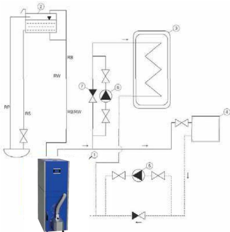
Rys. 4. Schemat poglądowy zabezpieczenia kotła DWOREK BIO COMPACT BLUE w układzie grzewczym otwartym, gdzie: 1 – kocioł, 2 – naczynie wzbiorcze (przelewowe), 3 – zasobnik c.w.u., 4 – obieg grzewczy, 5 – pompa c.o. (obiegowa), 6 – pompa c.w.u. (obiegowa), 7 – zawór różnicowy, RO – rura odpowietrzająca, RS – rura sygnalizacyjna, RB – rura bezpieczeństwa, RW – rura wzbiorcza, RP – rura przelewowa
