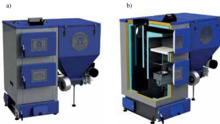
Rys. 1. Kocioł DWOREK ZPS EKO BLUE, gdzie: a) widok ogólny, b) przekrój przez kocioł
