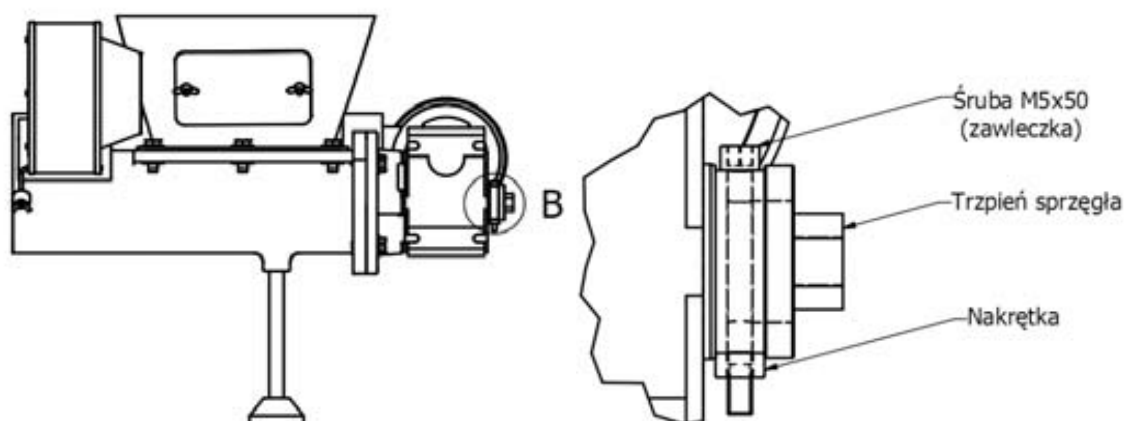
Rys. 8 Sposób montażu zawleczki motoreduktora ze ślimakiem
