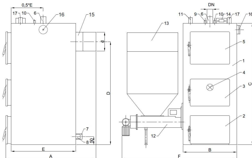
Rys.1. Kocioł „PRESTIGE-VR3”
