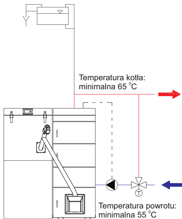
Ochrona powrotu zaworem termostatycznym
